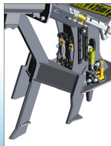
Sub-soilingverktyg för markberedning.
