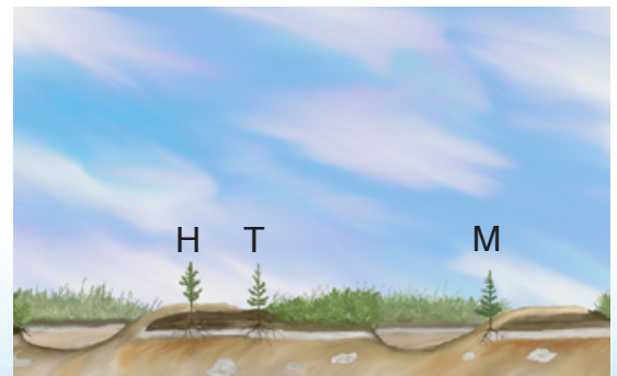
Bracke M24.a skapar planteringsställen med omvänd torva (T), mineraljordshög på omvänd torva (H) samt mineraljordshög på mineraljord (M).
