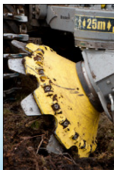
Tallrikar med utbytbara tänder.
