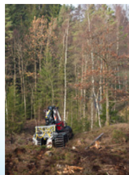
Bracke M24.a på en medelstor skotare ger ett mycket bra markberedningsresultat på alla högläggningsmarker.
