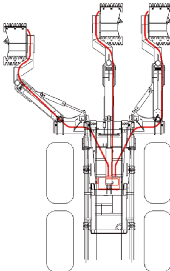
S35.a monteras på ett markberedningsaggregat och fröna matas ut i slangar till såddbädden. Individuella matarhjul kontrollerar flödet av frön till varje såddkanal.
